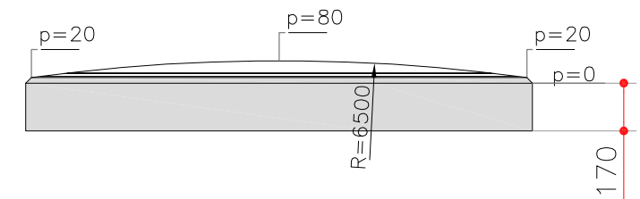
Doorsnede X'-X'
