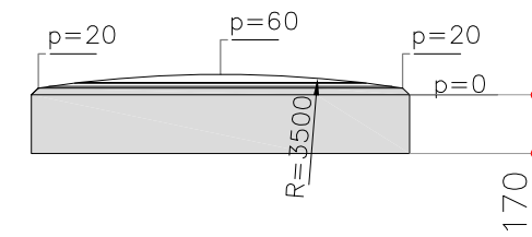
Doorsnede X''-X''
