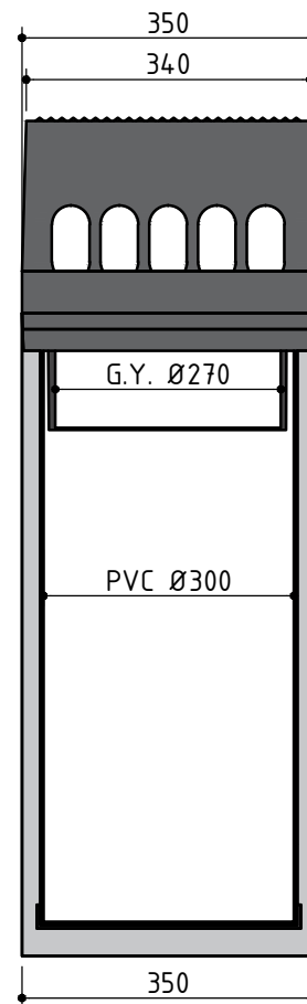
DOORSNEDE B-B
